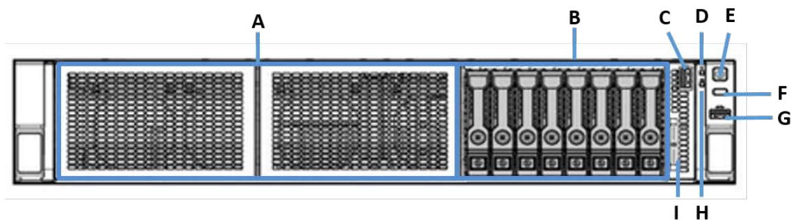
8x 2.5 型ドライブモデル正面図
