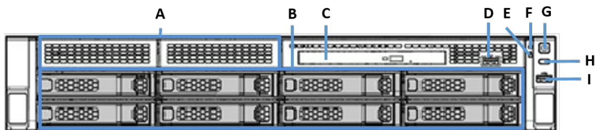
8x 3.5 型ドライブモデル正面図
