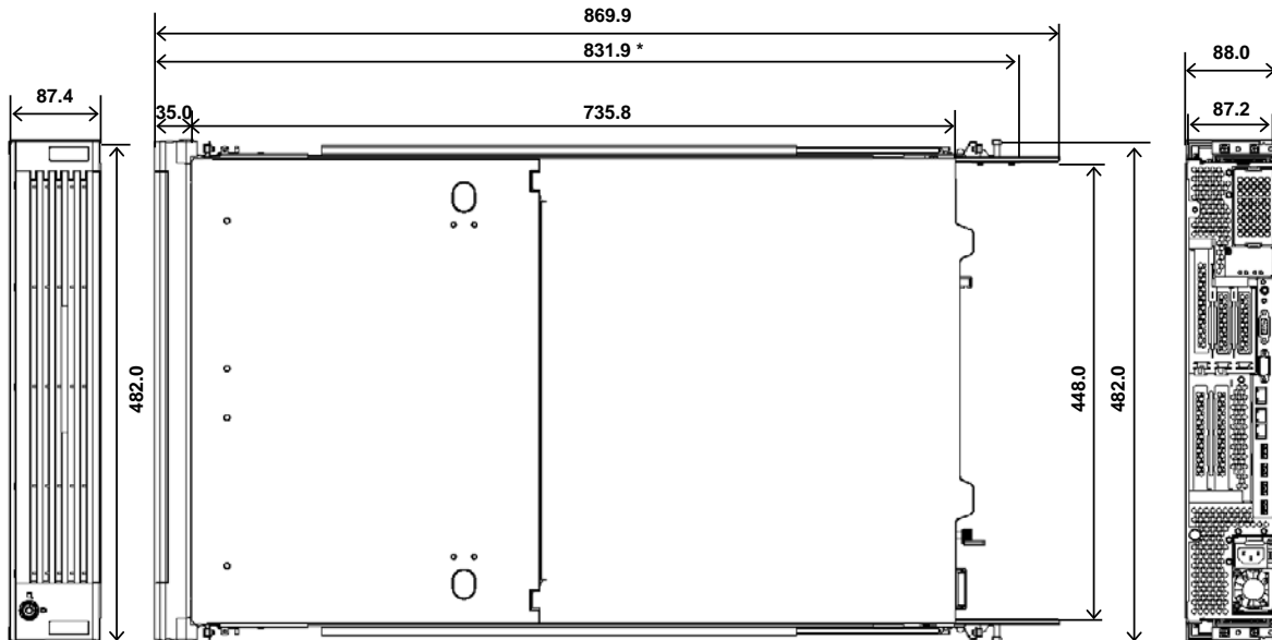
電源ユニット(450W), 電源ユニット(800W)搭載時 (単位: mm)
