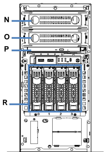
フロントベゼルを開いた状態 3.5 型 HDD ケージ(TN8154-79T)実装時
