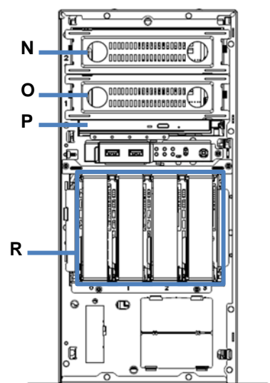
フロントベゼルを開いた状態 3.5 型 Fixed HDD ケージ(TN8154-81T)実装時
